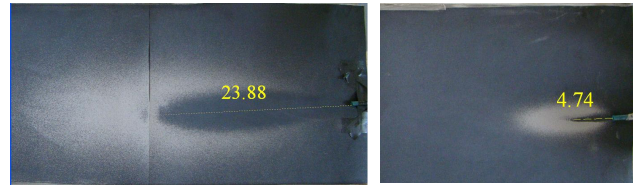
Figura 6. Distância (em mm) alcançada pelo jato de partículas com silo do alimentador modelo PM-PF-10 fechado (à esquerda.) e aberto (à direita), sob a mesma regulagem de vazão de gás (5 l/min, Ar)
