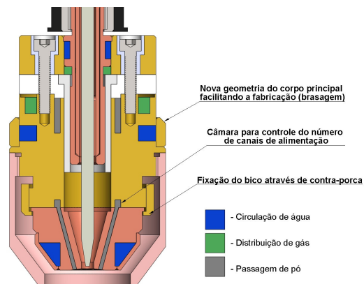
Figura 22. Inovações no projeto da tocha PTA-P
