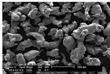
Figura 2. Pó metálico 316L atomizado em água
