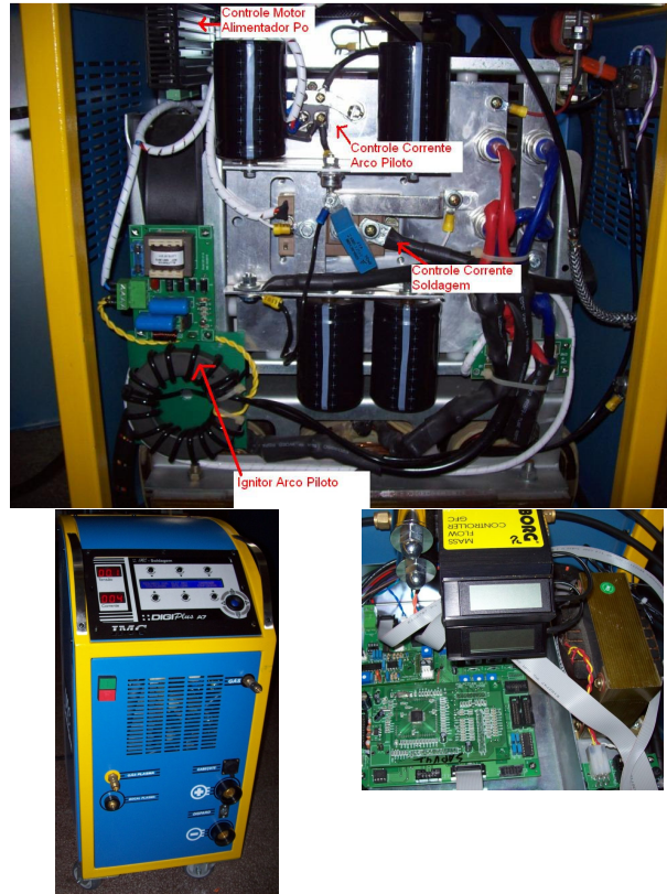
Figura 15. Sistema de Soldagem PTA-P dedicado
