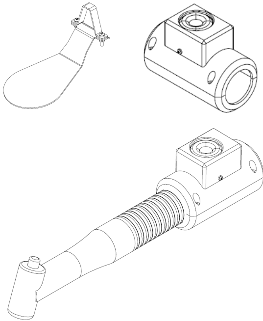
Figura 23. Proteção manual e unidade de regulagem de parâmetros de soldagem anexada à tocha (isolada e montada)
