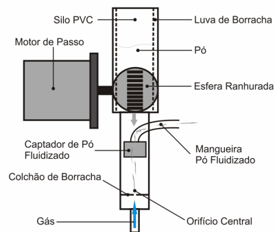
Figura 7. Esquema do ADP-2 com silo aberto
