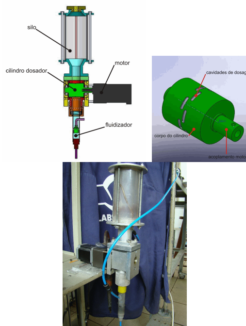
Figura 11. Modelo em CAD do ADP-2, cilindro dosador e ADP-2 montado
