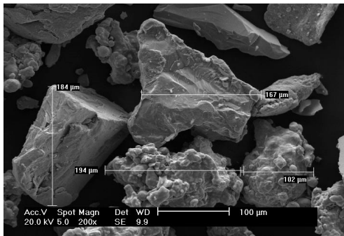
Figura 4. Morfologia da liga LO3* (mistura de pós triturados)
