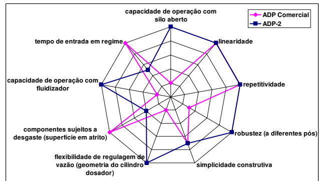
Figura 13. Gráfico em rede comparativo entre os ADPs investigados
