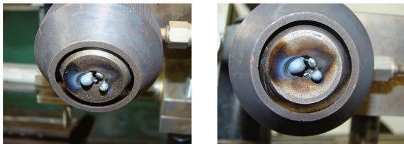
Figura 20. Tocha com injeção interna de pó e seus canais entupidos por material aderido (corrente de soldagem: 190 A, taxa de alimentação de pó: 17,5 g/min)
