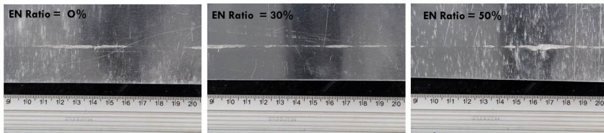
Figura 88 - Versos das chapas para corpos de prova referentes aos EN Ratios de 0%, 30% e 50%. MIG Pulsado CA (OTC DW-300, gap = 1,5 mm).
