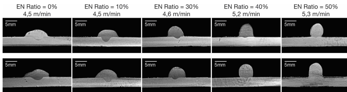
Figura 96 - Macrografias para MIG/MAG Pulsado CA (OTC DW-300). Chapas soldadas com diferentes EN Ratios e velocidade de alimentação de arame variando conforme a EN Ratio.
