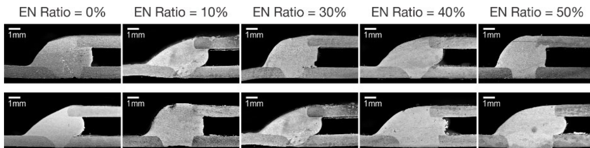
Figura 86 - Macrografias para MIG/MAG Pulsado CA (OTC DW-300, gap = 1,5 mm). Juntas soldadas com diferentes EN Ratios.
