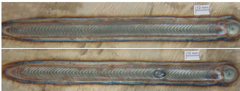
Figura 38 - Cordões de solda com switch back pulsado de acordo com a Tabela 6
