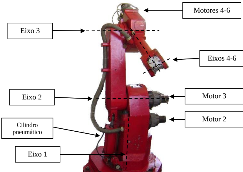
Figura 16 – Estrutura do braço robótico
