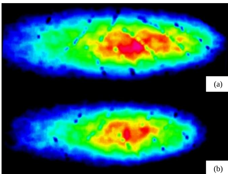
Figura 43 – Distribuição de calor no lado oposto ao soldado, para movimentação linear (a) e switch back (b)
