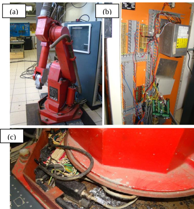
Figura 15- Fotos tiradas em maio de 2013 demonstrando a situação precária do robô: braço robótico (a), painel eletroeletrônico (b) e base do braço robótico (c)
