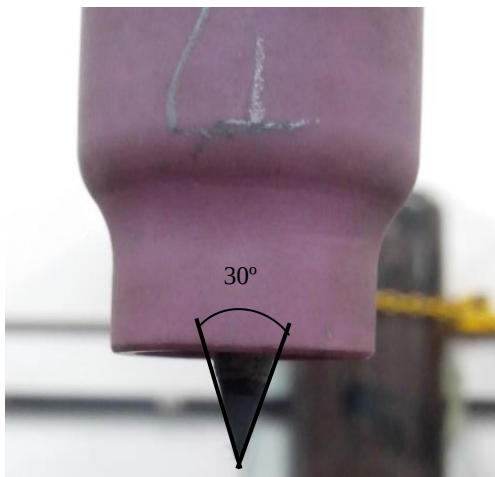
Figura 35 - Afiação do eletrodo utilizada em todos os ensaios
