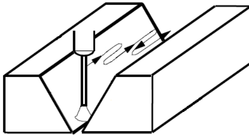
Figura 11 – Oscilação switch back [17]
