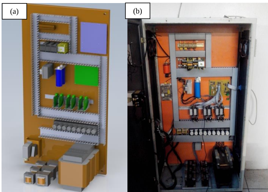
Figura 24 - Gabinete eletro-eletrônico modelado no SolidWorks (a) e gabinete após o retrofitting (b)
