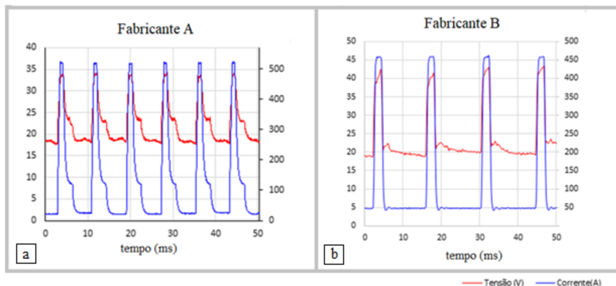
Figura 5. Oscilogramas para os programas sinérgicos dos Fabricante A e Fabricante B com V_a = 4,1\text{m/min} e gás de proteção \text{Ar-18\%CO}_2 .
