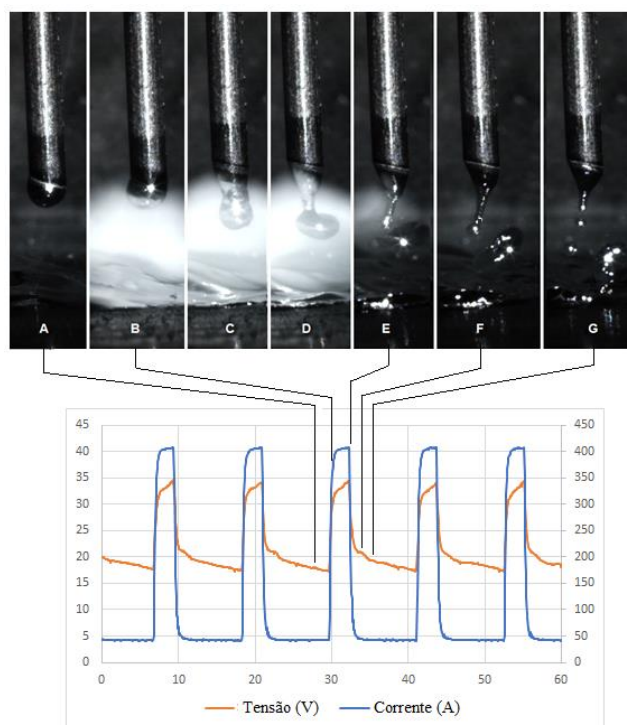
Figura 7. Validação do expoente de 1,37 via filmagem de alta velocidade. Ensaio 3.1 da Tabela 5.
