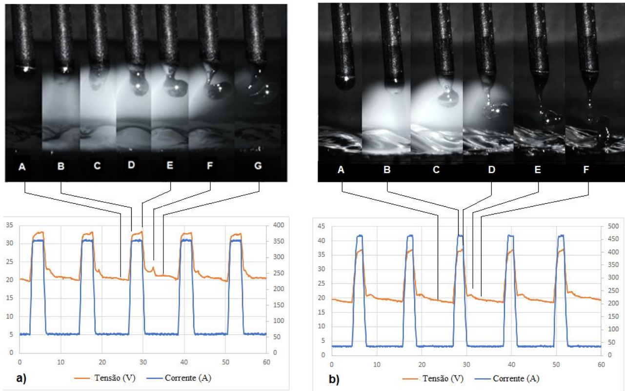
Figura 6. Filmagem em alta velocidade para ensaio da Tabela 4 a) cod.1.6 b) cod. 2.1.
