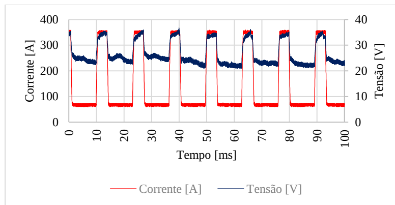
Figura 4. Oscilogramas obtidos para o conjunto de parâmetros cód. 2.
